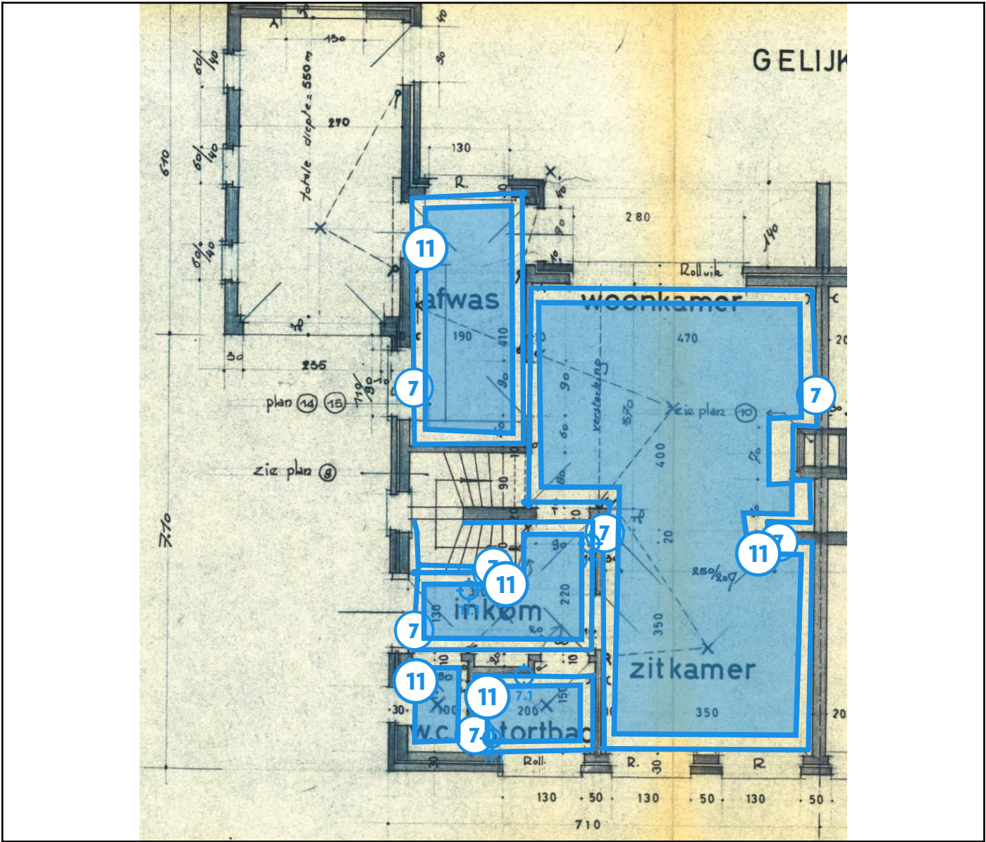
Legende van plan 1.7: Gelijkvloers - pleisterwerk
