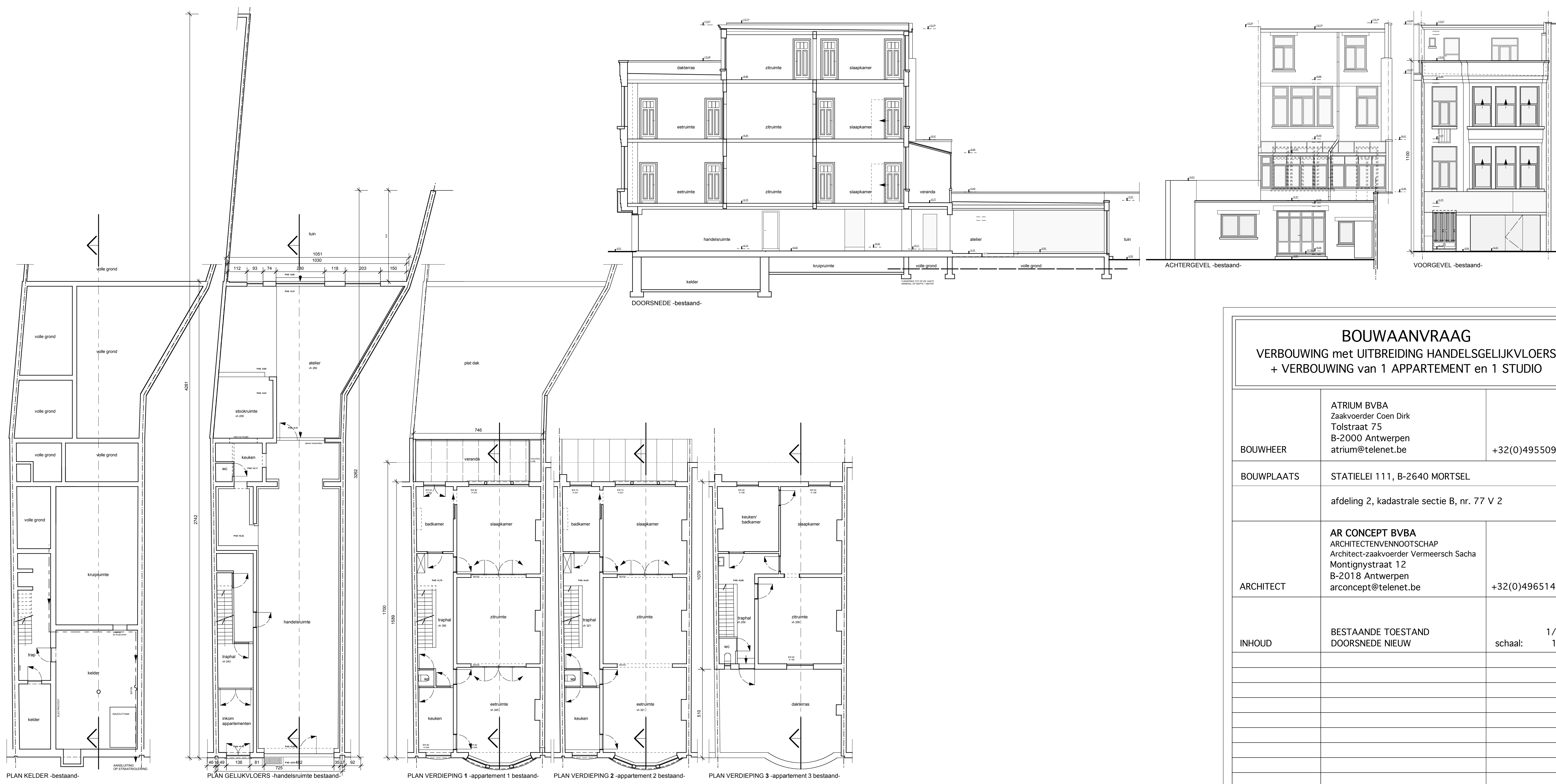
DOORSNEDE -nieuw-
