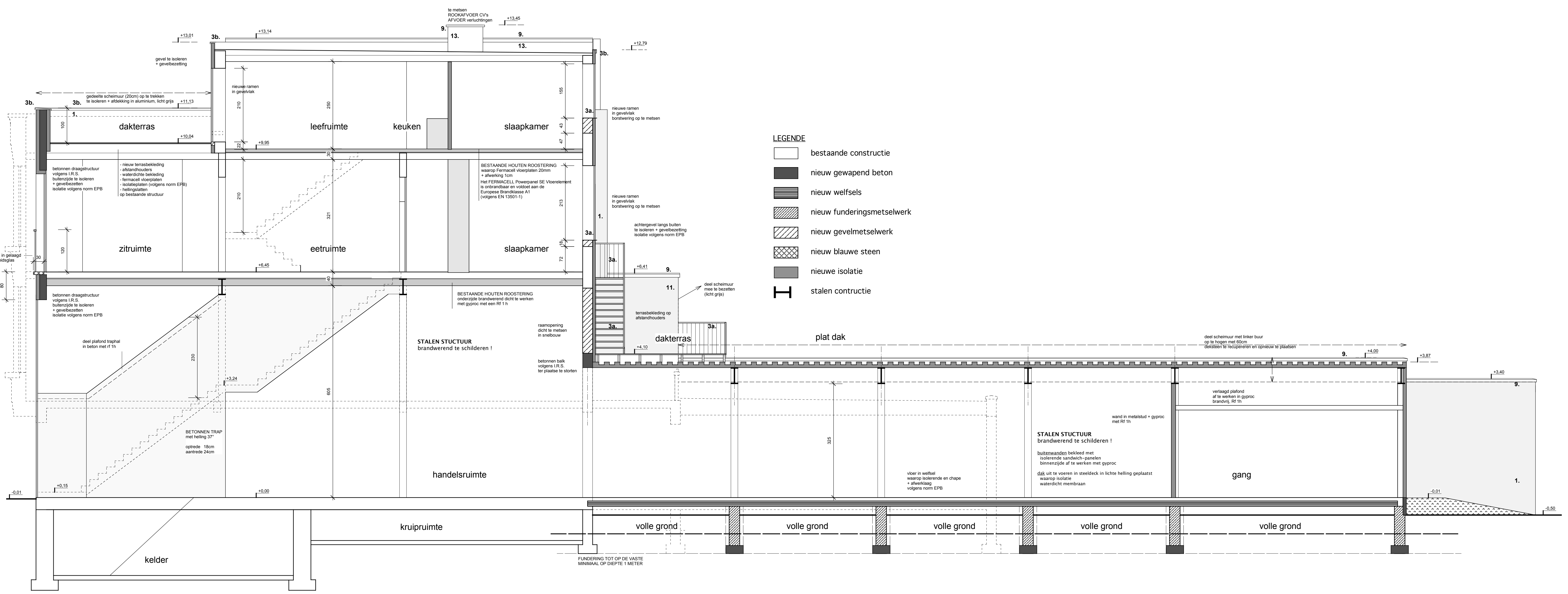
DOORSNEDE -nieuw-
